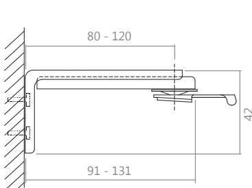
wysięgnik regulowany 80/120
