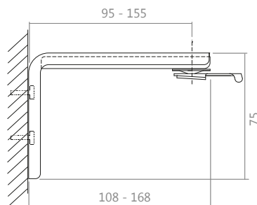
wysięgnik regulowany 95/155
