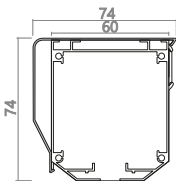
Przekrój rynny
